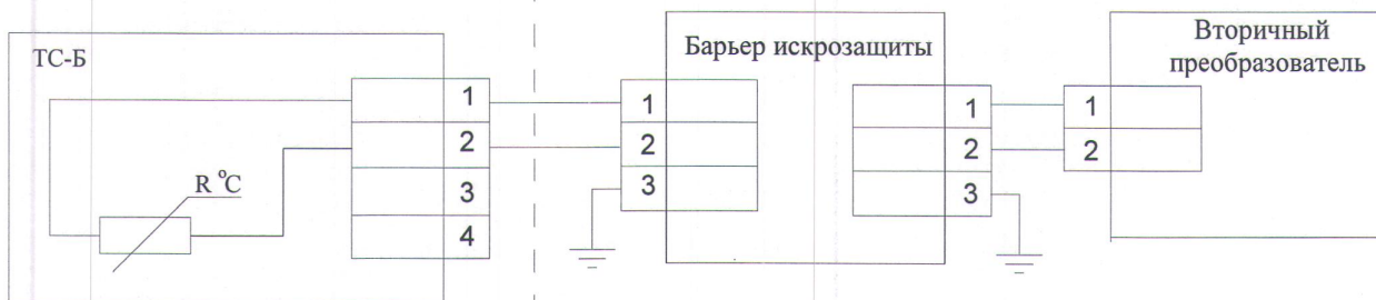
Рисунок В.3 Схема подключения взрывозащищенного ТС-Б, с видом взрывозащиты «искробезопасная цепь» уровня «ia», с 2-х проводной схемой подключения к вторичному преобразователю (устройству индикации) .
