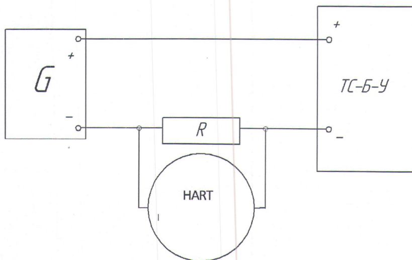
Рисунок 2.6.1 - Схема подключения внешних цепей ТС-Б-У с выходным сигналом (4-20) мА и совмещенным протоколом HART
