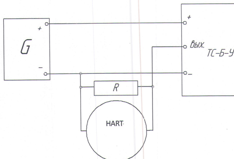
Рисунок 2.6.2 - Схема подключения внешних цепей ТС-Б-У с выходным сигналом (0-20) мА и (0-5) мА и совмещенным протоколом HART
