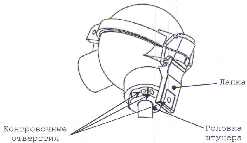
Рисунок Г.2 - Расположение контрольных отверстий термопреобразователя с клеммной головкой исполнения Д.
