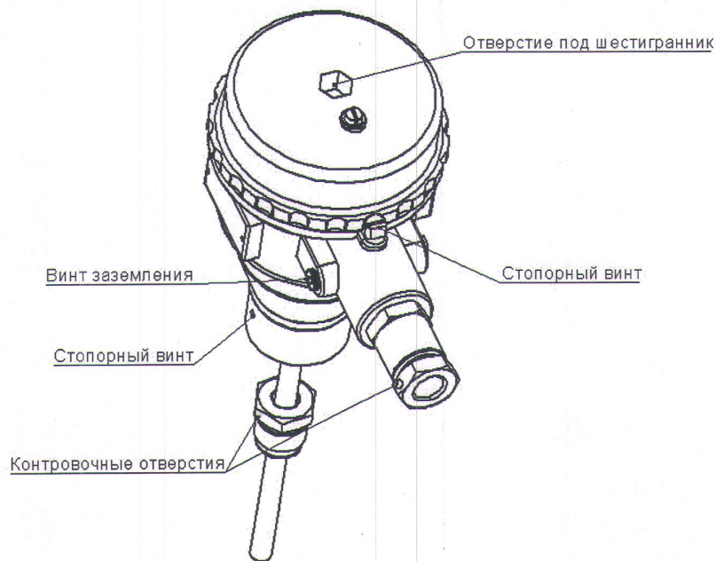
Рисунок Г.4 - Расположение контровочных отверстий термопреобразователя с клеммной головкой исполнения М.
