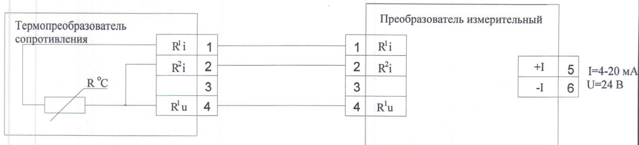
Преобразователь измерительный нумерация указана условно
