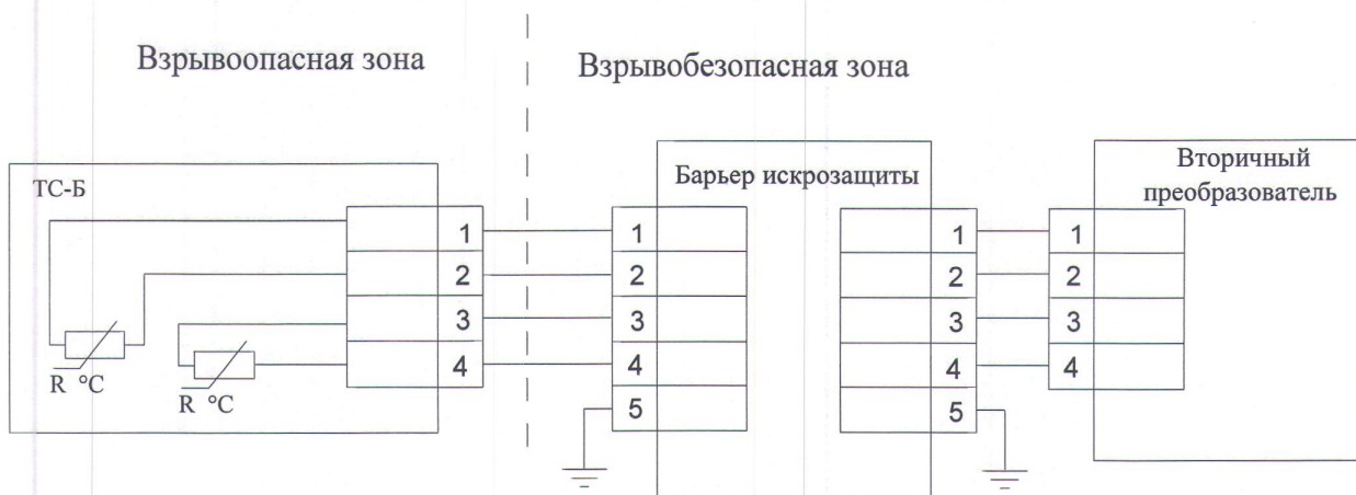
Рисунок В.6 Схема подключения взрывозащищенного ТС-В-Р, с видом взрывозащиты «искробезопасная цепь» уровня «ia», с двумя чувствительными элементами, с 2-х проводной схемой подключения к вторичному преобразователю (устройству индикации).
