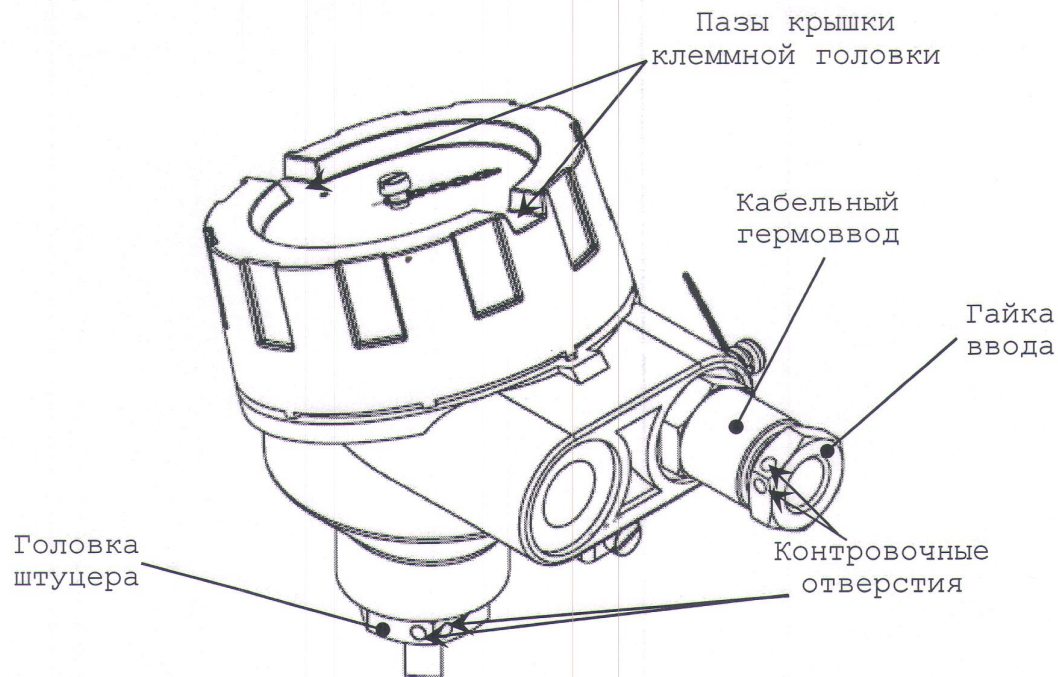
Рисунок Г.3 - Расположение контровочных отверстий термопреобразователя с клеммной головкой исполнения М2.
