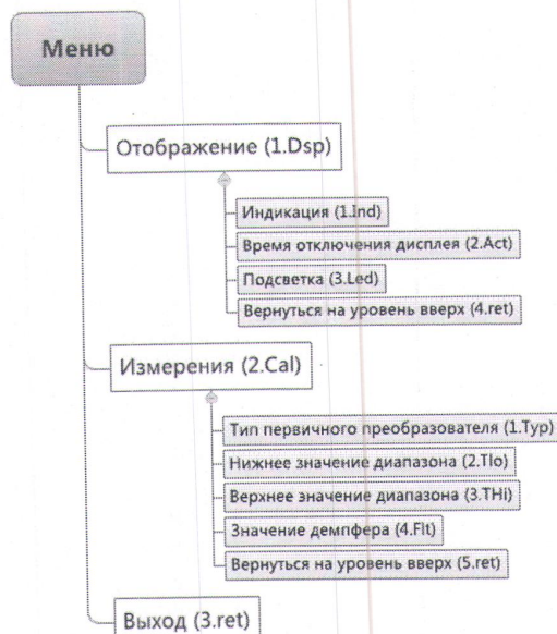
Рисунок 1 – меню индикатора с преобразователем температуры
