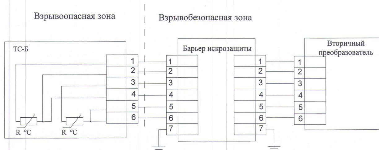
Рисунок В.7 Схема подключения взрывозащищенного ТС-В-Р, с видом взрывозащиты «искробезопасная цепь» уровня «ia», с двумя чувствительными элементами, с 3-х проводной схемой подключения к вторичному преобразователю (устройству индикации).
