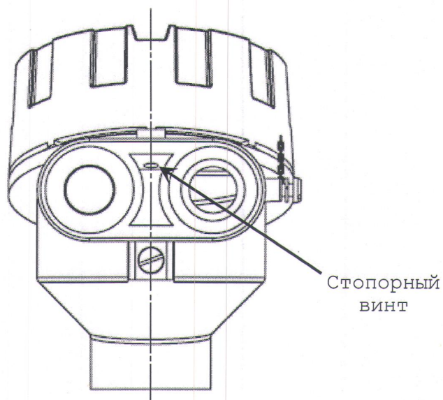
Рисунок Г.1 - Расположение стопорного винта в клеммной головке исполнения М2
